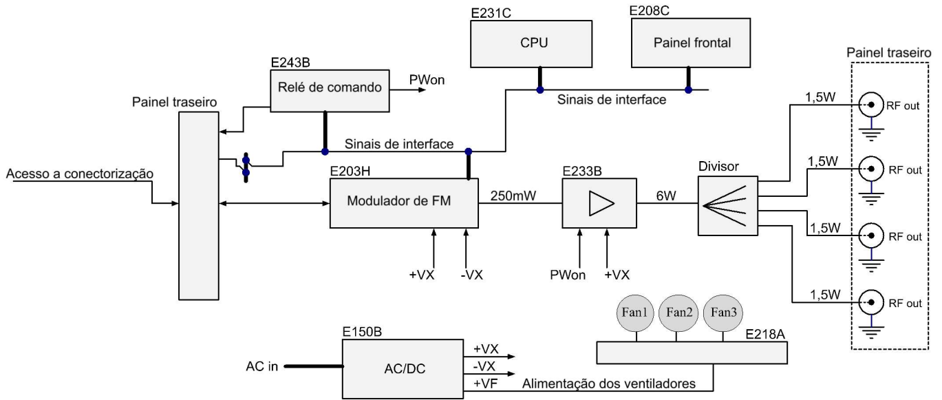
Figura 9: Diagrama em blocos MC124S/E
