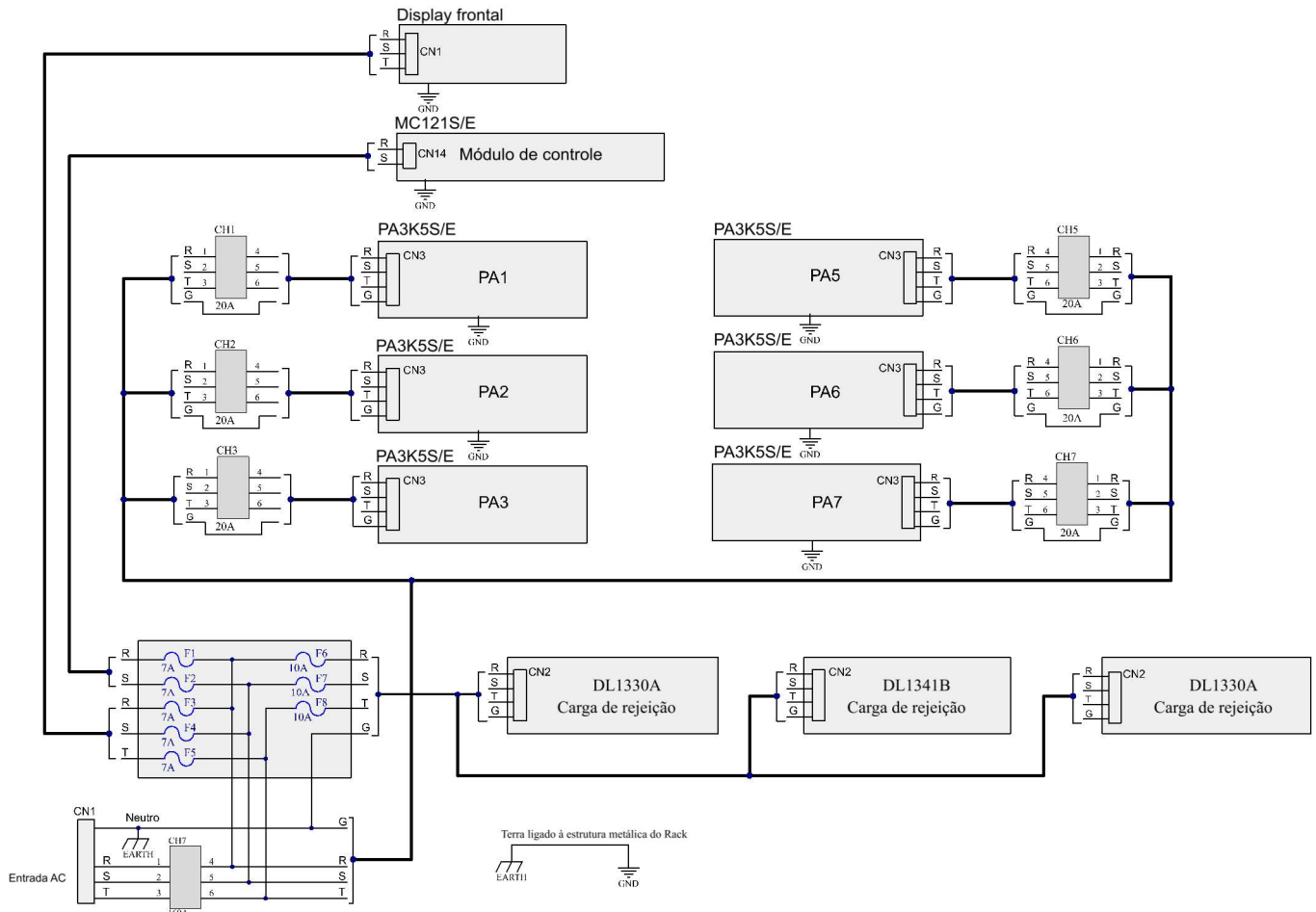
Figura 2: Alimentação AC
