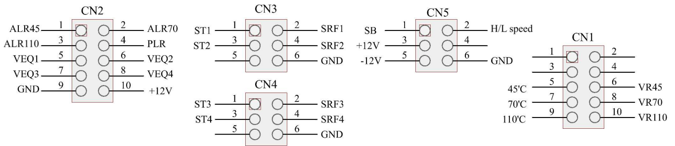
Figura 49: Conectores E279A
