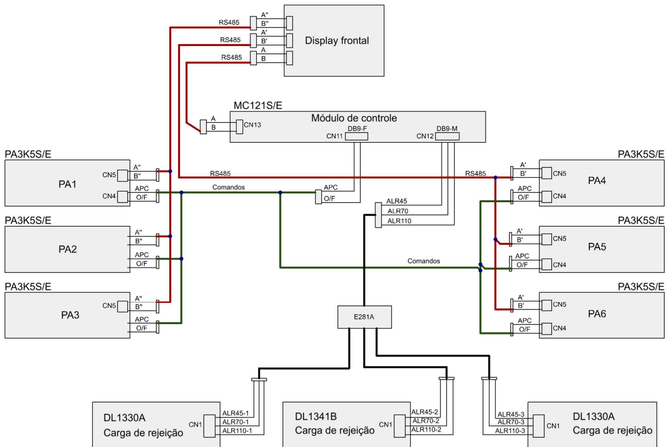
Figura 3: Controle
