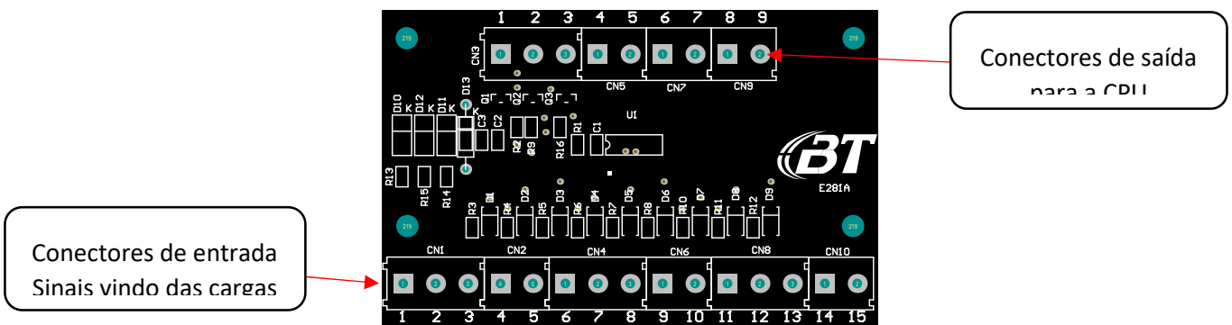
Figura 5: PCI E281A
