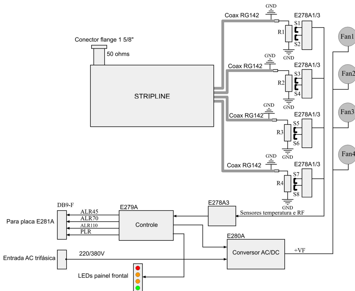
Figura 47: Diagrama em blocos DL1330S/E
