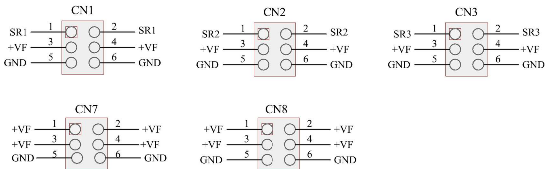
Figura 33: Conexões E159E
