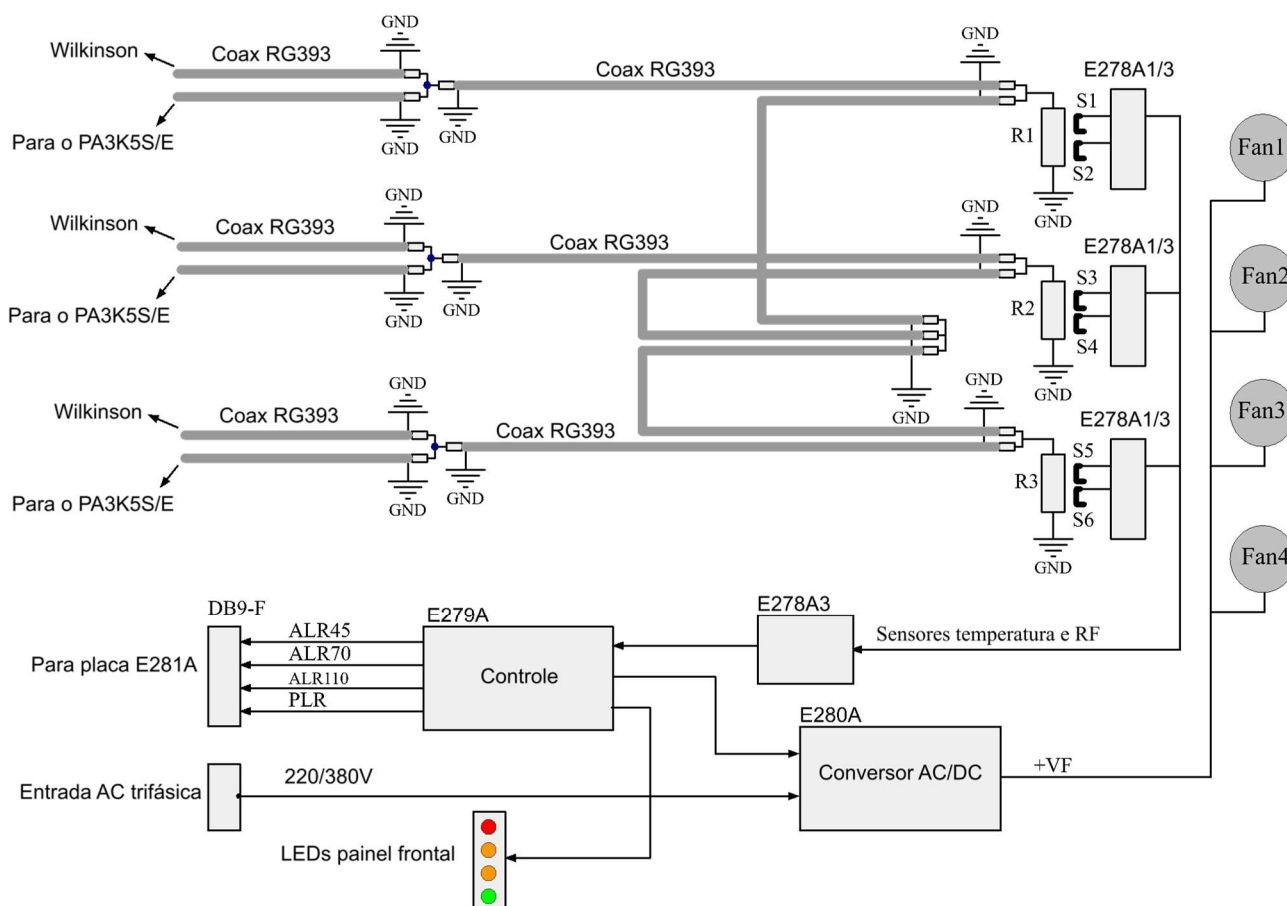
Figura 38: Diagrama em blocos DL1330S/E
