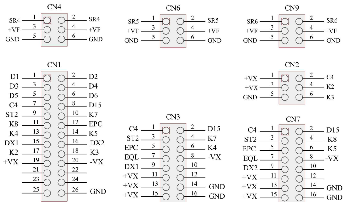
Figura 31: Conexões E158E
