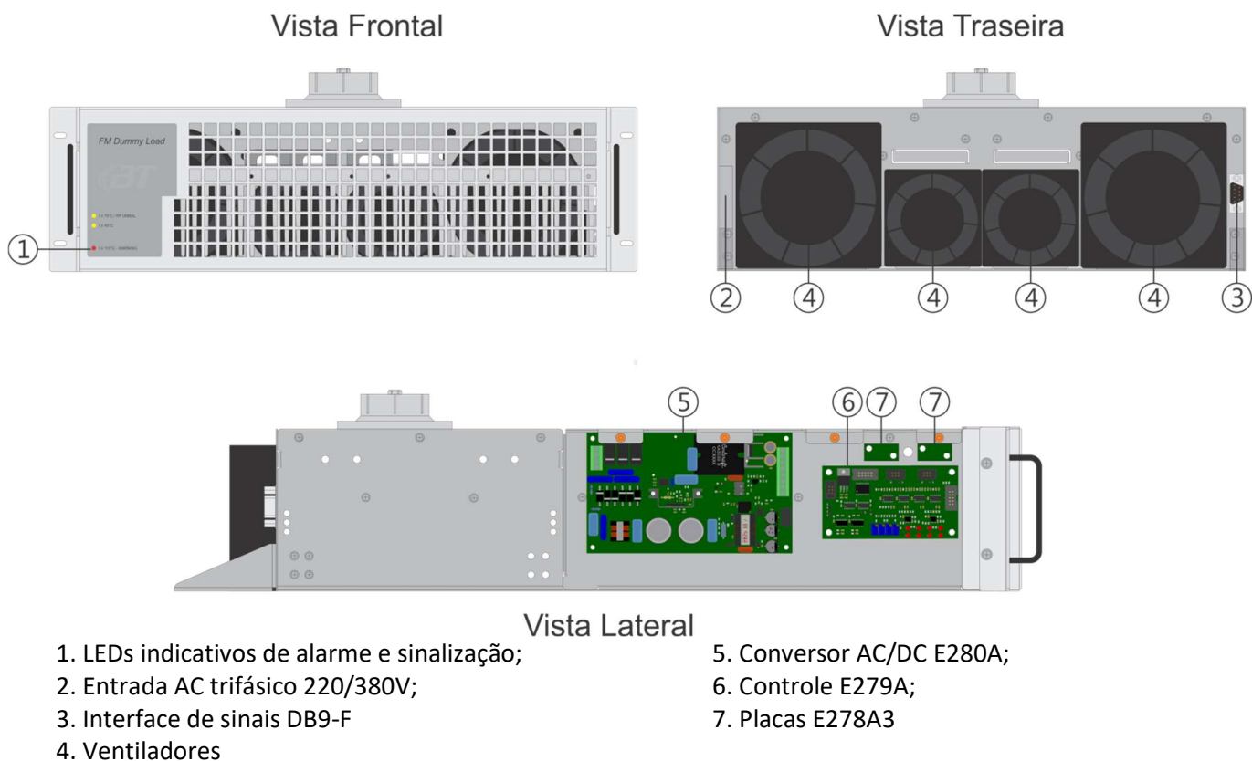
Figura 46: Vistas frontais e traseira DL1330S/E
